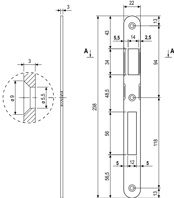
A-A section
